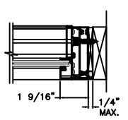
④ JAMB FIXED FLUSH ADAPTER
